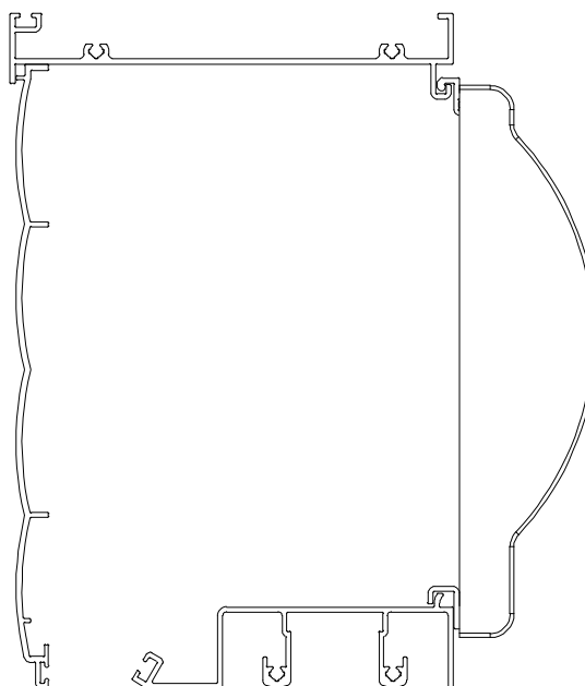
Instalação - escala 1:2
