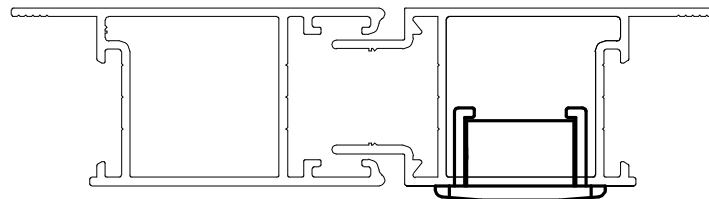
Instalação - escala 1:1
