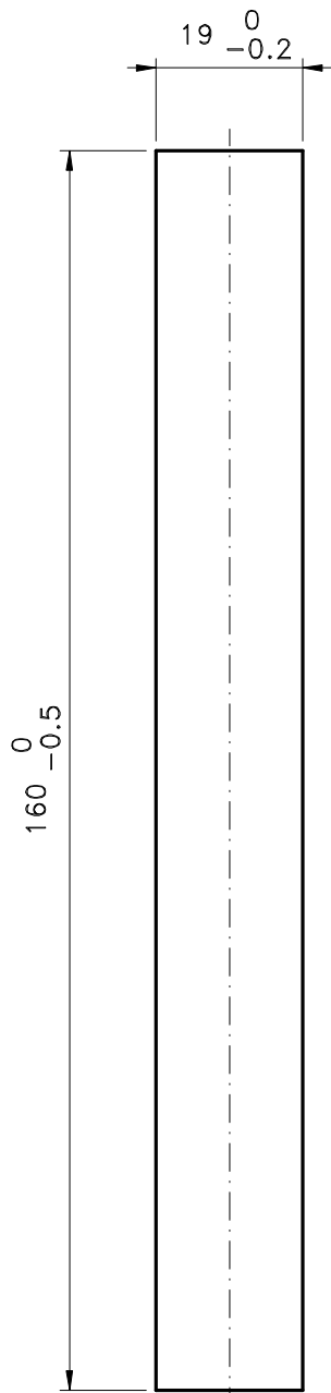
Usinagem - escala 1:1
