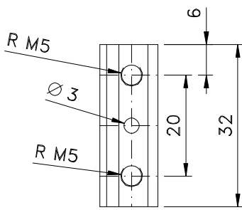
Vistas - escala 1:1
