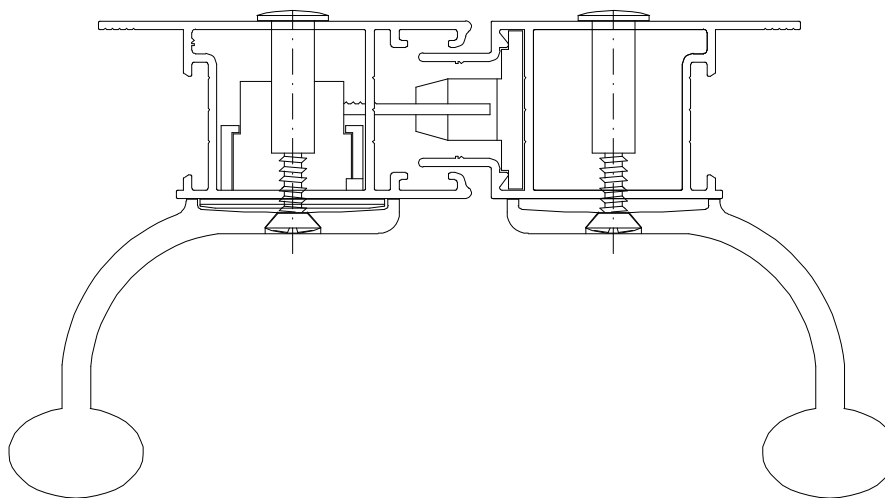
Instalação - escala 1:1
