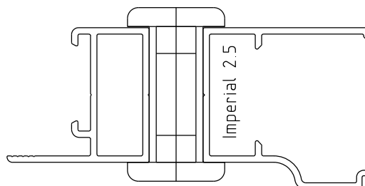
Instalação - escala 1:1
