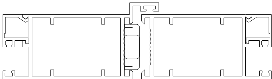
Instalação - escala 1:1
