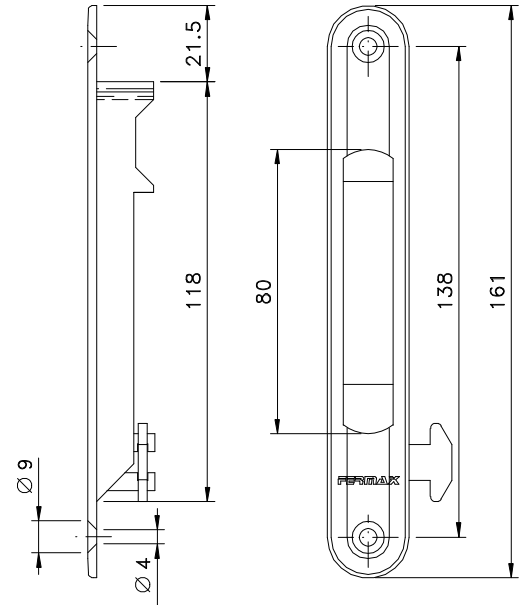
Vistas - escala 1:2
