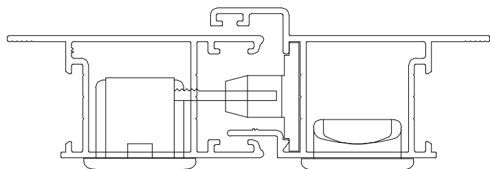
Instalação - escala 1:1
