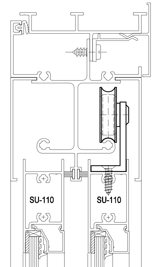
Instalação - escala 1:1
