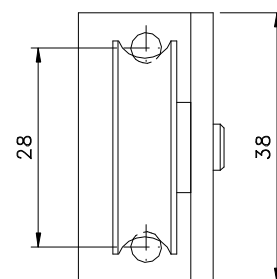
Vistas - escala 1:1
