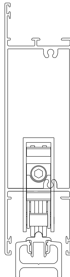
Instalação - escala 1:1
