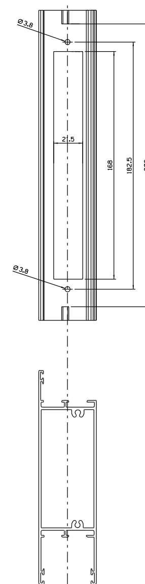
Usinagem - escala 1:2
