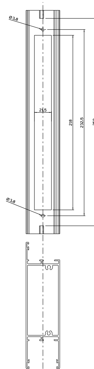
Usiagem - escala 1:2
