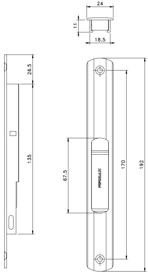
Vista - escala 1:2
