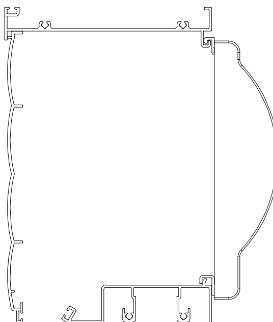
Instalação - escala 1:2
