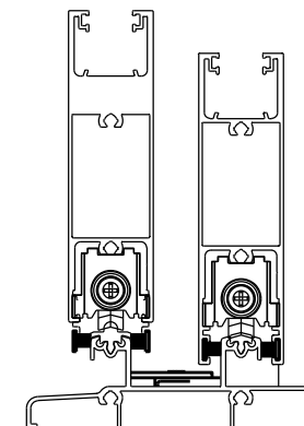
CHROMA
