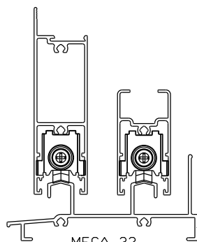
MEGA 32
