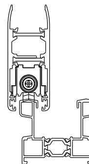
TERA_AURA55C
