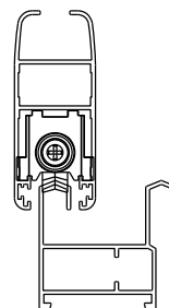
TERA_AURA40
