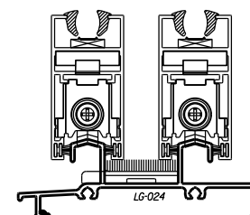
MAGNAPLUS
