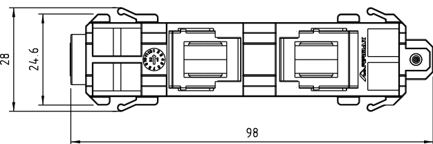
Vistas - escala 1:1
