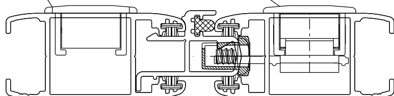
Instala**o - escala 1:1
