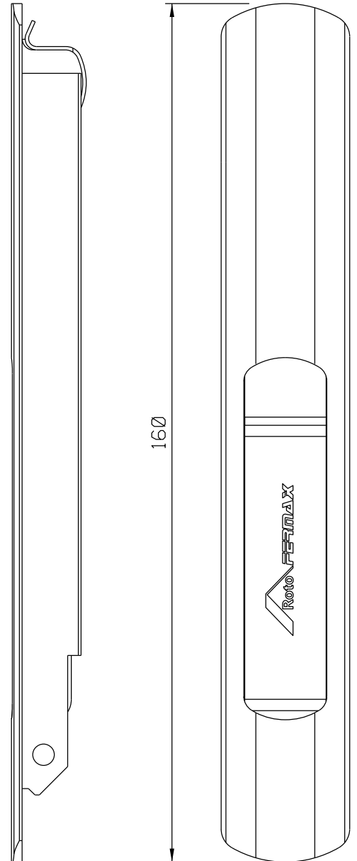
Vistas - escala 1:1
