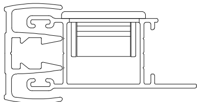
Instalação - escala 1:1
