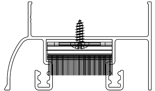
Vistas - escala 1:1
