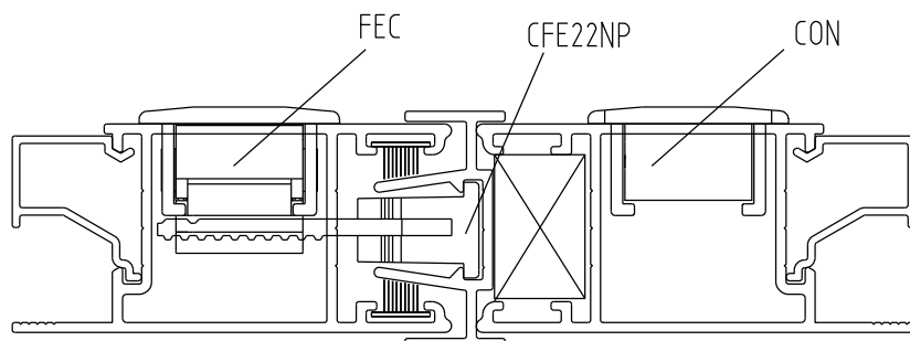
Instalação - escala 1:1
