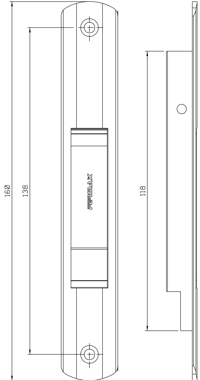
Vistas - escala 1:1
