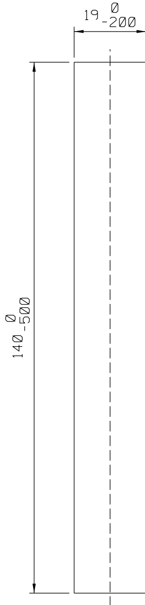
Usinagem - escala 1:1
