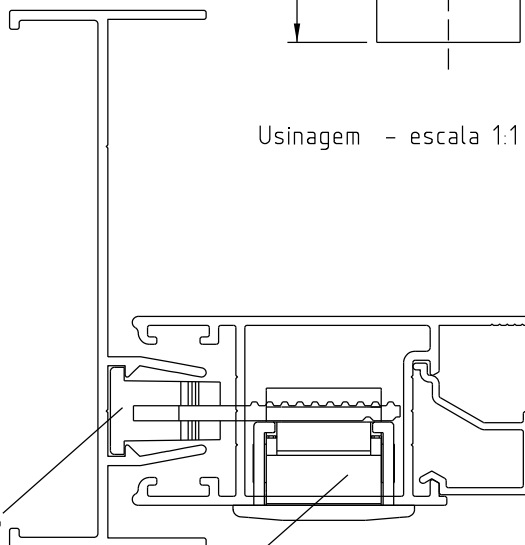
Instalação - escala 1:1
