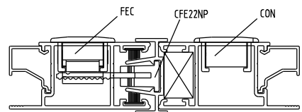
Instalação - escala 1:2
