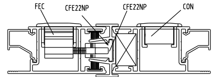
Instalação - escala 1:2
