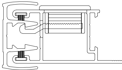
Instalação - escala 1:1
