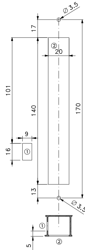
Usinagem - escala 1:2
