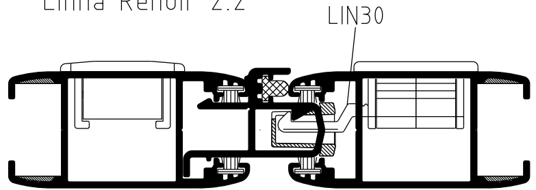
INSTALAÇÃO 1:1
