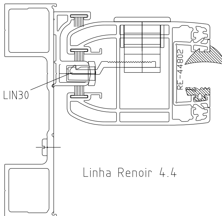
INSTALAÇÃO 1:1
