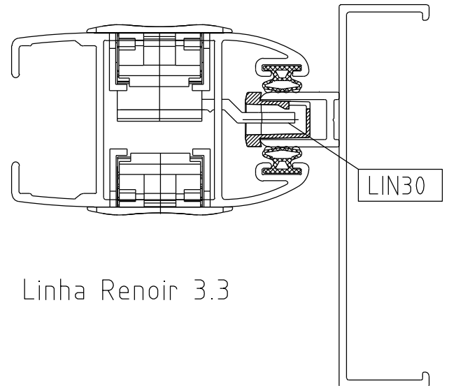
ESCALA 1:1
