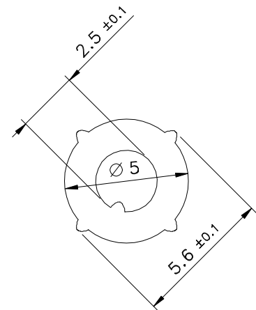
Vista – escala 5:1
