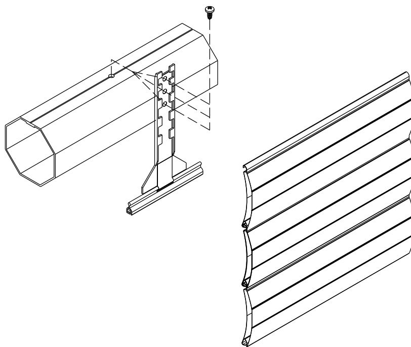
DETALHE DE APLICAÇÃO - sem escala
