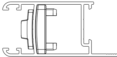
Instalação - escala 1:1
