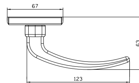
VISTAS Escala 1:2
