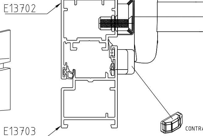
INSTALAÇÃO Escala 1:1
