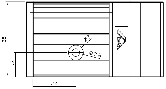
Vistas - escala 1:2
