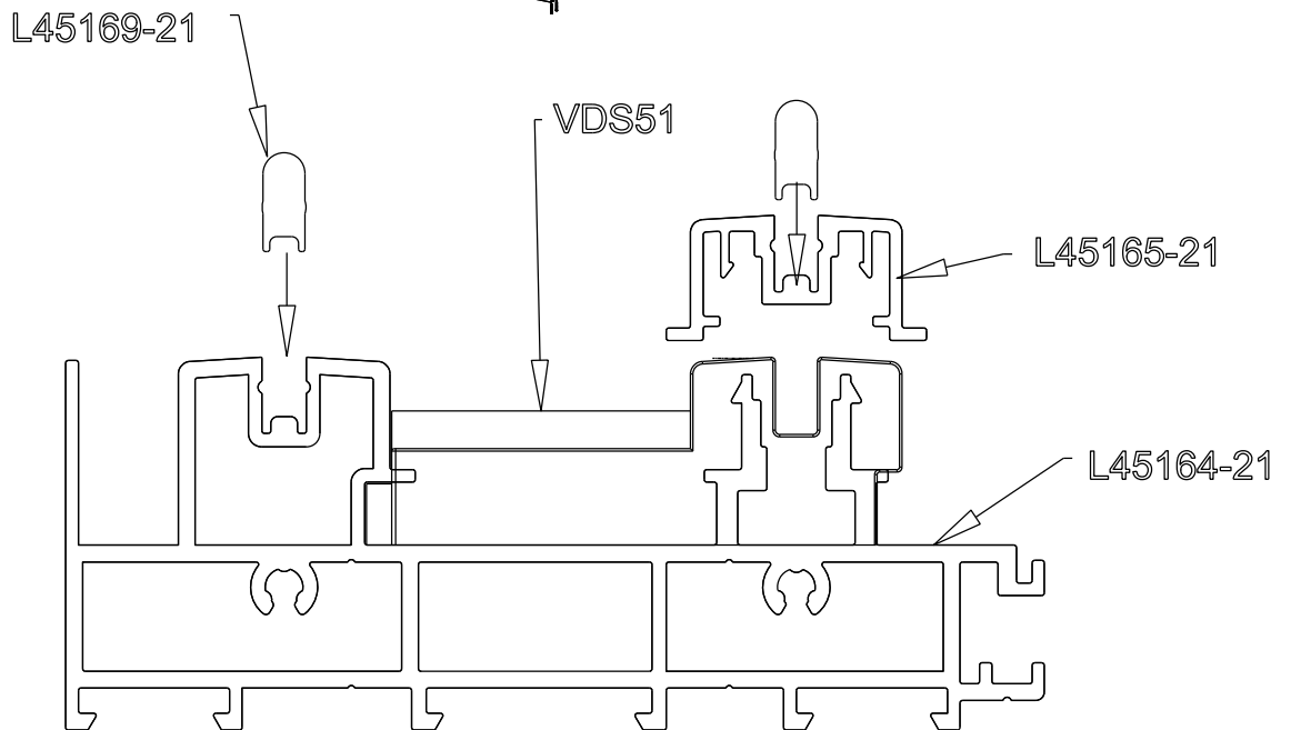
Instalação - escala 1:1
