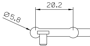
Vistas - escala 2:1
