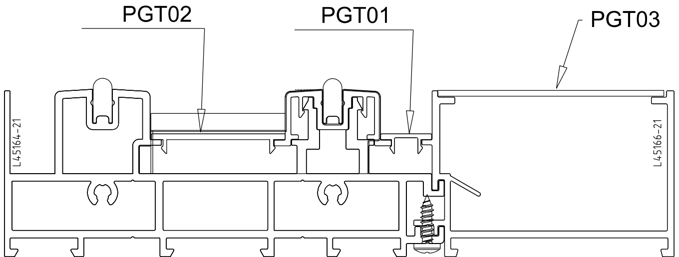
Vistas - escala 1:1
