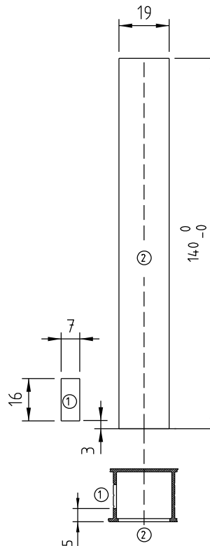
Usinagem - Escala 1:2
