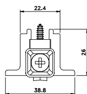
Vistas - escala 1:2
