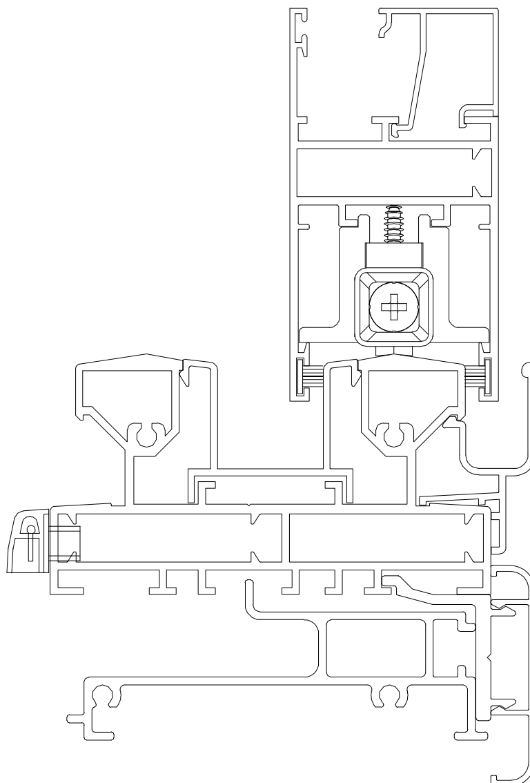
Instalação - escala 1:1
