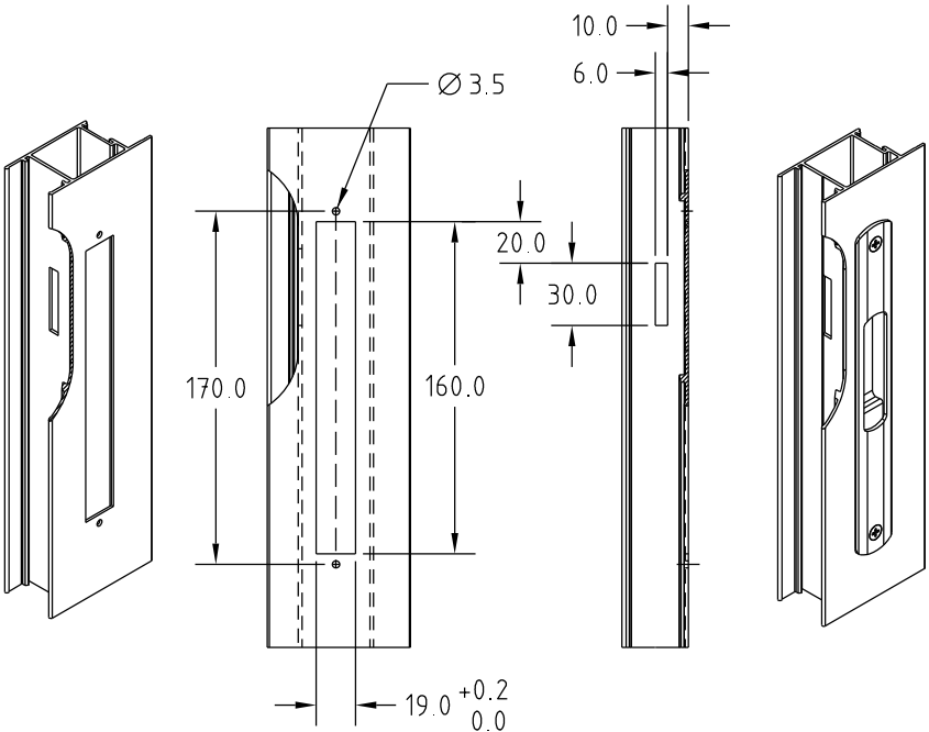
USINAGEM Escala 1:4
