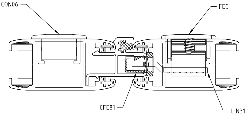
INSTALAÇÃO Linha RENOIR 2.2 SISTEMISTA CDA ESCALA 1:1
