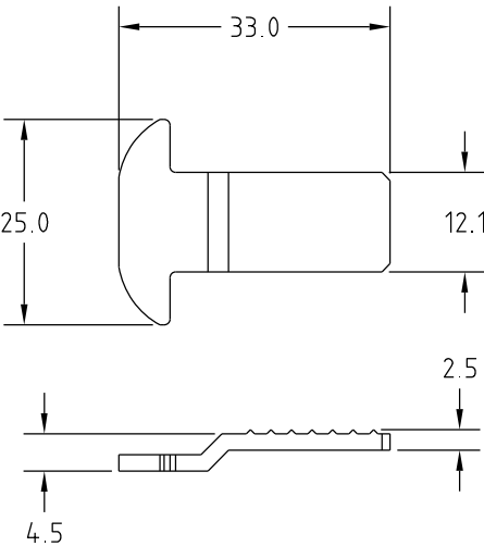
Vistas: Escala 1:1
