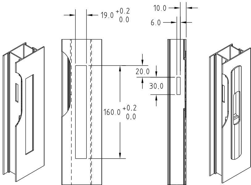
USINAGEM Escala 1:4
