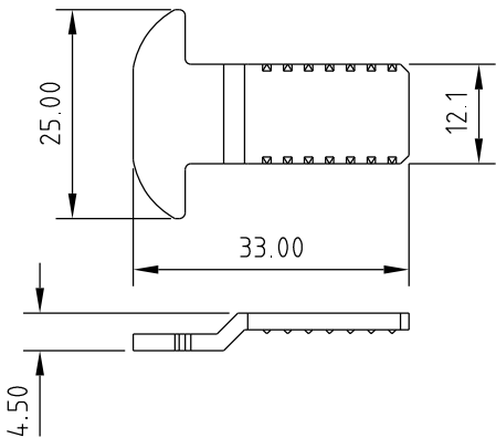
Vistas: Escala 1:1
