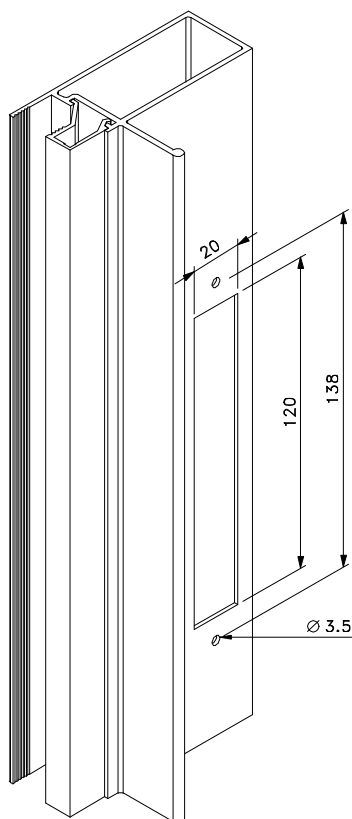
Usinagem - sem escala
