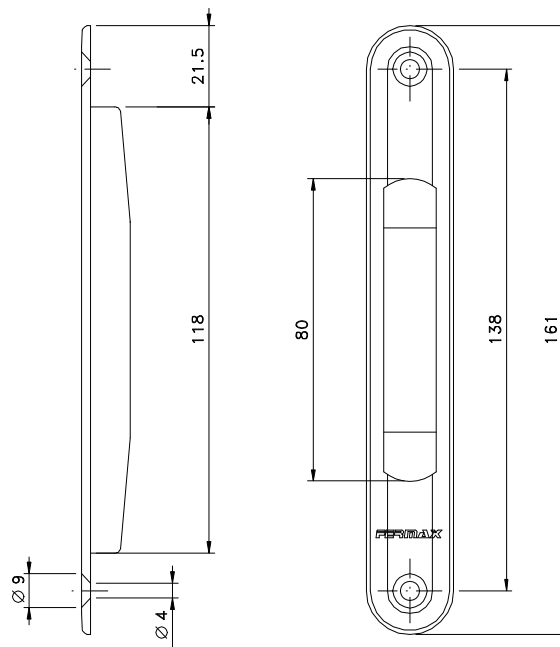
Vistas - escala 1:2
