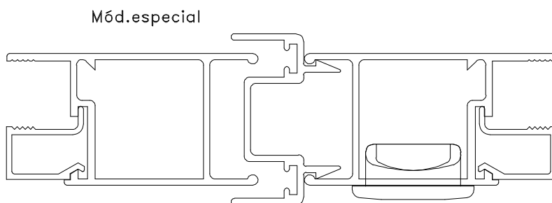
Instalação - escala 1:1
