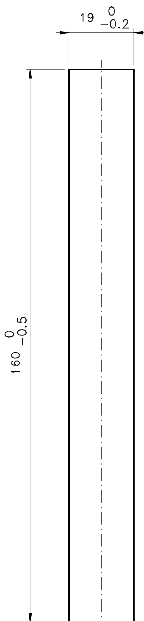
Usinagem — escala 1:1
