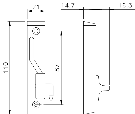
Vistas - escala 1:2
