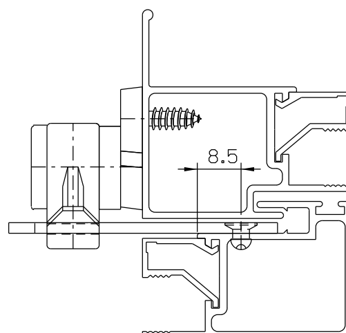
ESCALA 1:1
