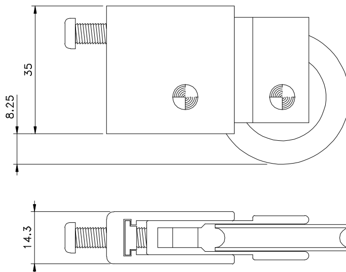
Vistas - escala 1:1
