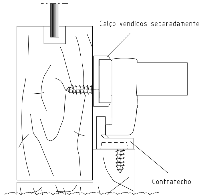
Instalação - escala 1:1
