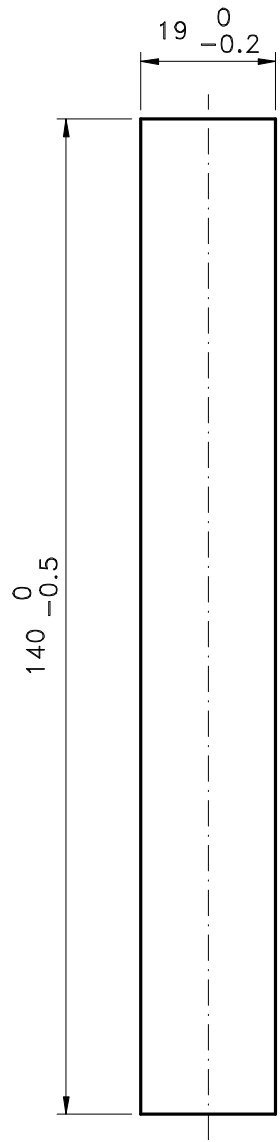
Usinagem - escala 1:1
