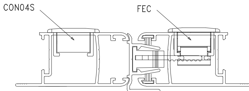
Instalação - escala 1:1
