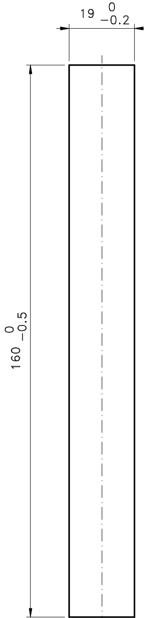
Usinagem - escala 1:1
