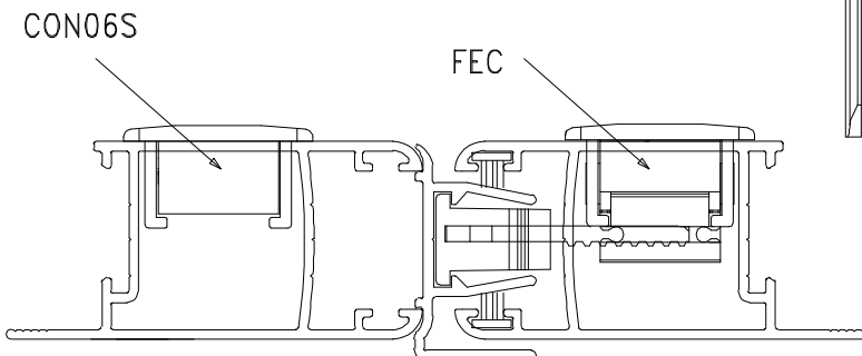
Instalação - escala 1:1
