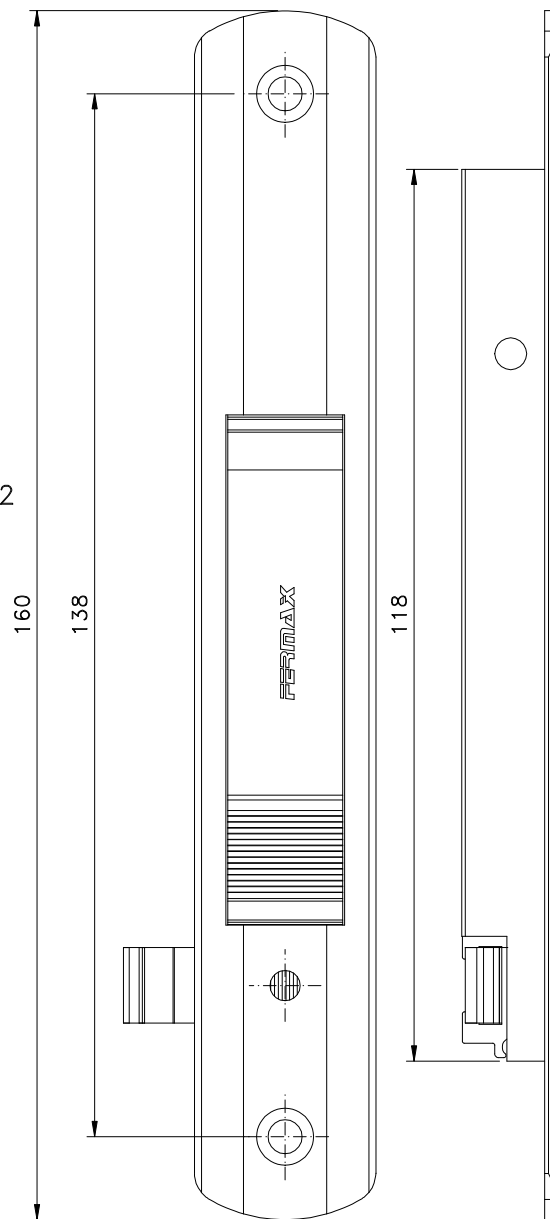
Vistas - escala 1:1
