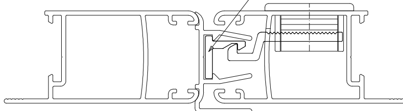
Instalação - escala 1:1
