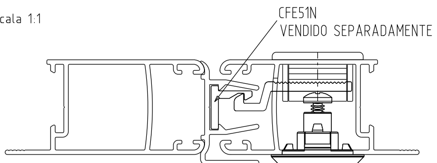
Instalação - escala 1:1
