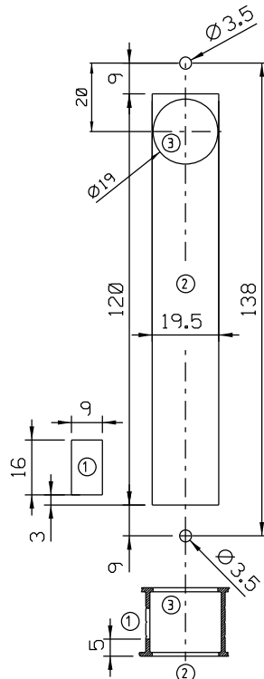
Usinagem - escala 1:2
