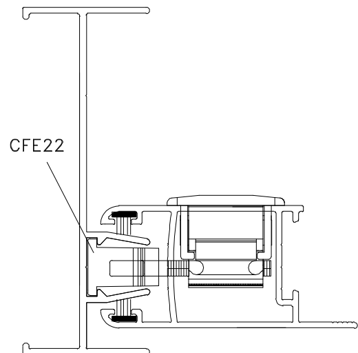
Vistas - escala 1:2
