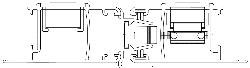
Instalação - escala 1:2
