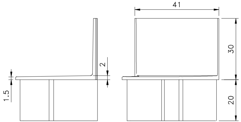
Vistas - escala 1:1
