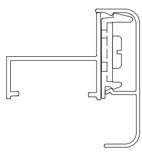
Instalação - escala 1:1
