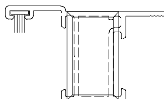
Instalação - escala 1:1
