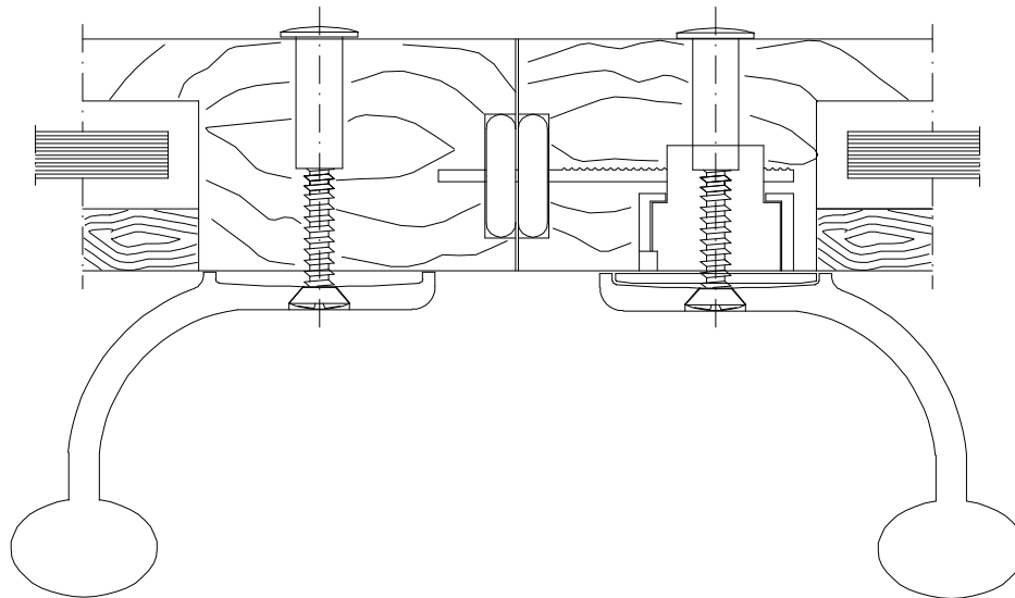
Instalação - escala 1:1
