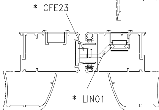
Usinagem - escala 1:1
